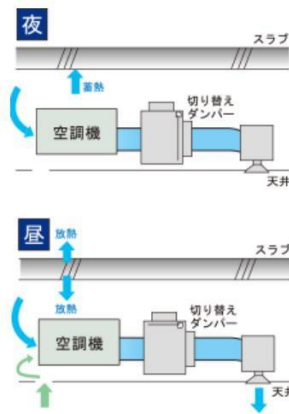
躯体蓄熱システム
